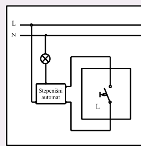
Taster svetla
