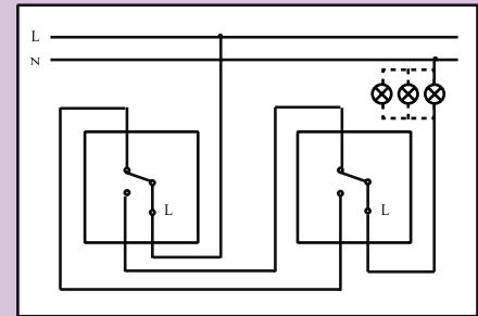
Naizmenična sklopka
