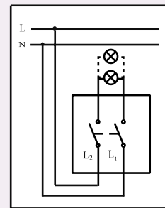
Dvopolna sklopka
