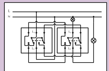
Dvostruka naizmenična sklopka
