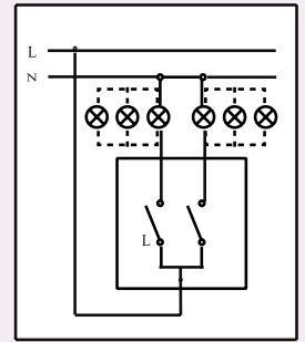
Serijska sklopka
