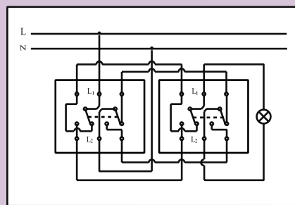
Dvopolna naizmenična sklopka
