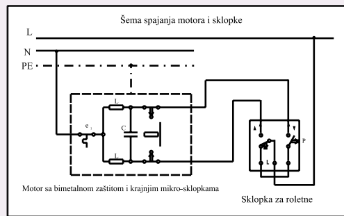
Taster za roletne i motor Šema veze
