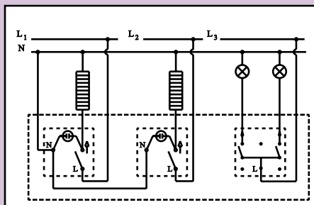
Vertikalna sklopka za kupatilo sa serijskom sklopkom
