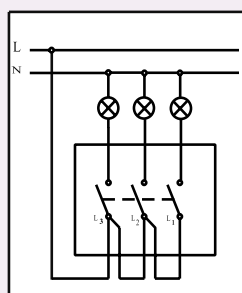
Tropolna sklopka
