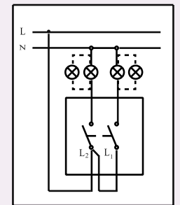
Dvopolna sklopka (drugi način veze)
