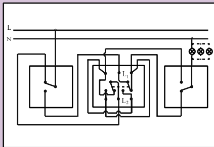
Unakrsna sklopka
