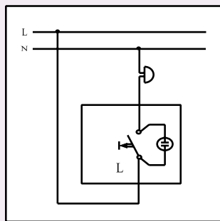
Taster zvona sa sig. sijalicom Taster SOS sa sig. sijalicom Taster sa pločicom za natpis i sig. sijalicom
