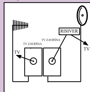
TV priključnica 2M završno - završna
