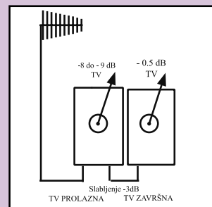
TV priključnica 2M prolazno - završna
