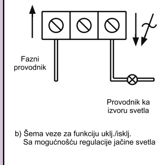
Regulator svetlosti sa potencijetrom
