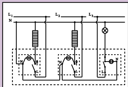
Vertikalna sklopka za kupatilo
