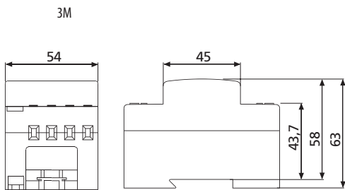
Signalno svjetlo 2 SS 220
